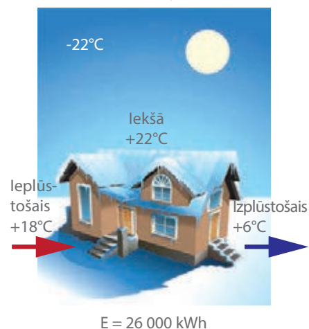
Risinājums ar plākšņu siltummaini
